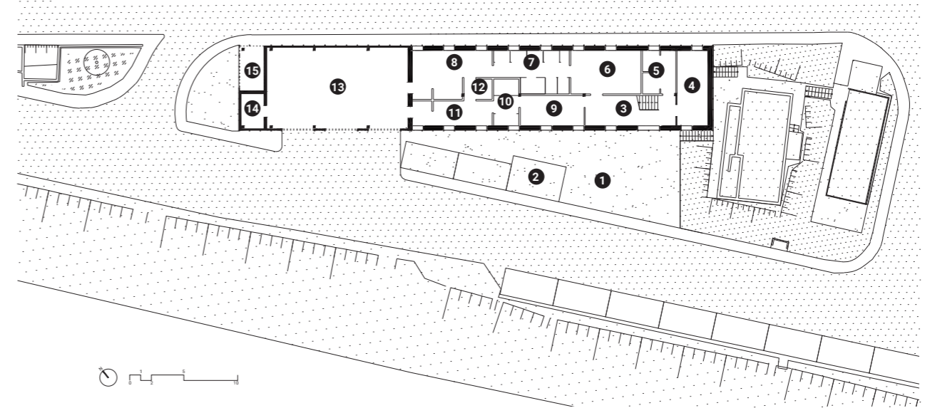
plan RDC
